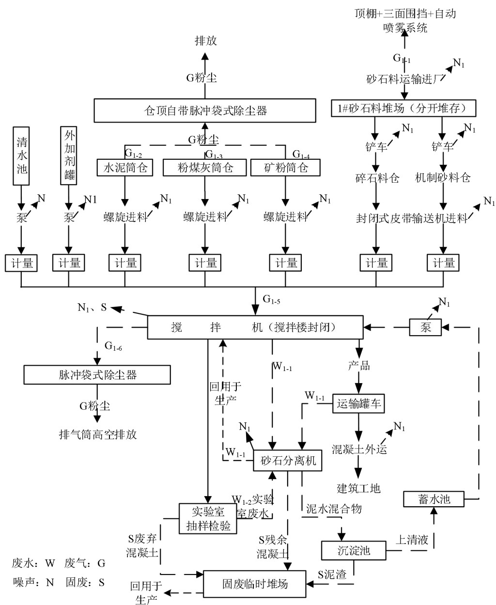
图2-4 商品混凝土生产工艺流程图
