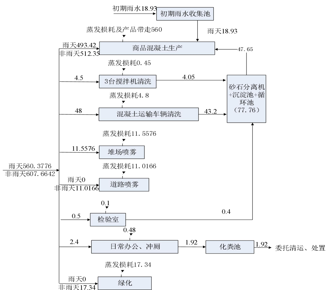
图 2-1 项目日水平衡示意图 单位: \text{m}^3/\text{d}
