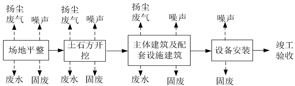
图 2-3 施工期工艺流程及产污环节示意图
