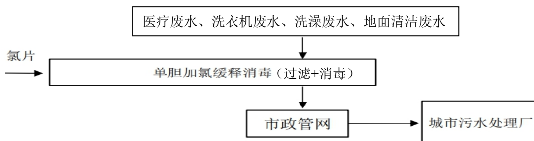
图 4-3 一体化污水处理设备工艺流程
