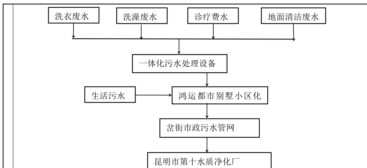
图 4-2 医院污水收集、处理流程
