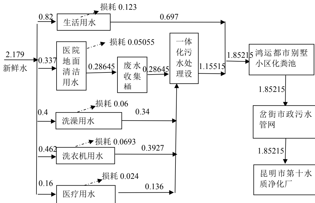
图 4-1 项目水平衡图 单位: m³/d
