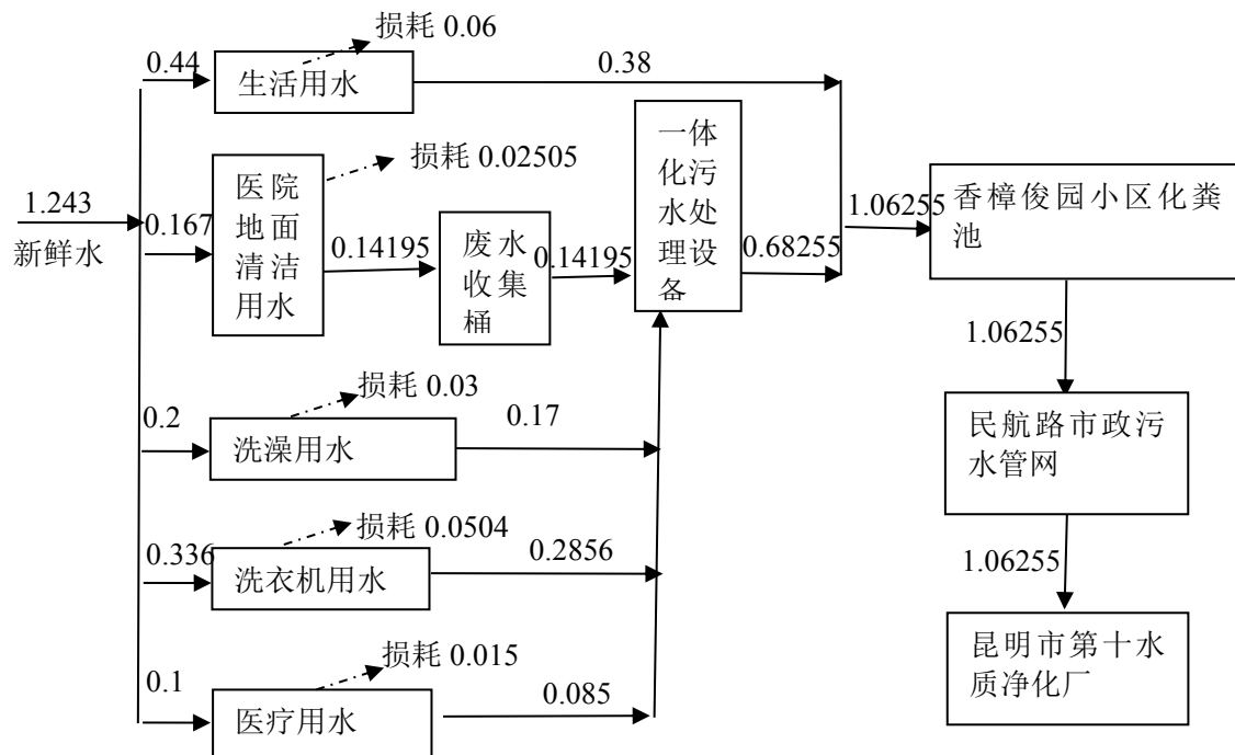
图 4-1 项目水平衡图 单位: \text{m}^3/\text{d}
