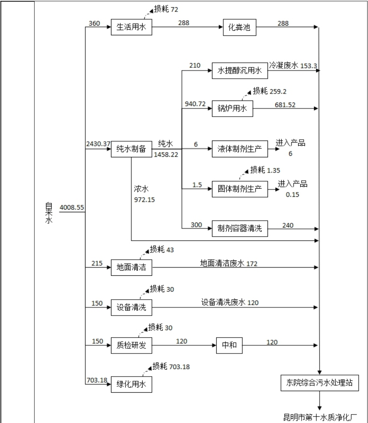
图 2-1 项目水量平衡图 (单位: m³/a)
