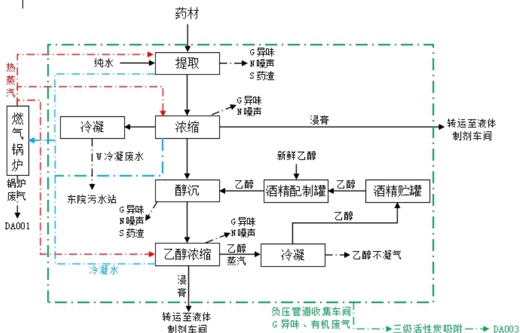
图 2-2 提取车间工艺流程及产污节点图
