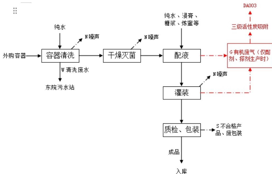
图 2-3 液体制剂生产工艺流程及产污节点图
