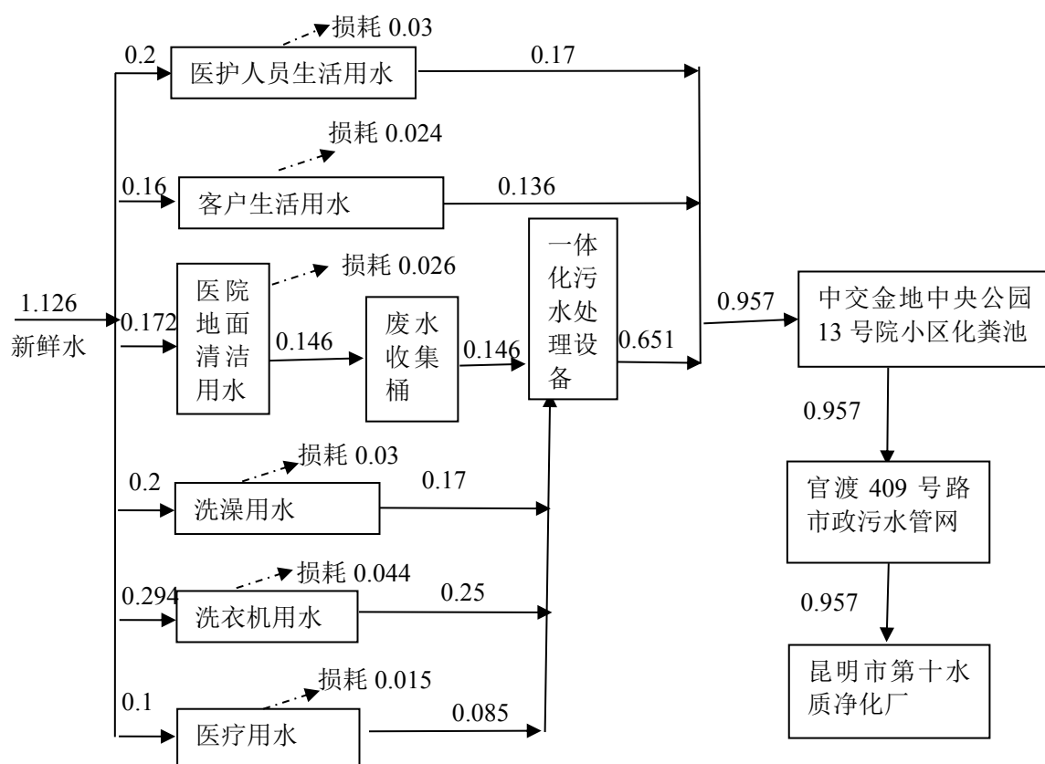
图 4-1 项目水平衡图 单位：m³/d
