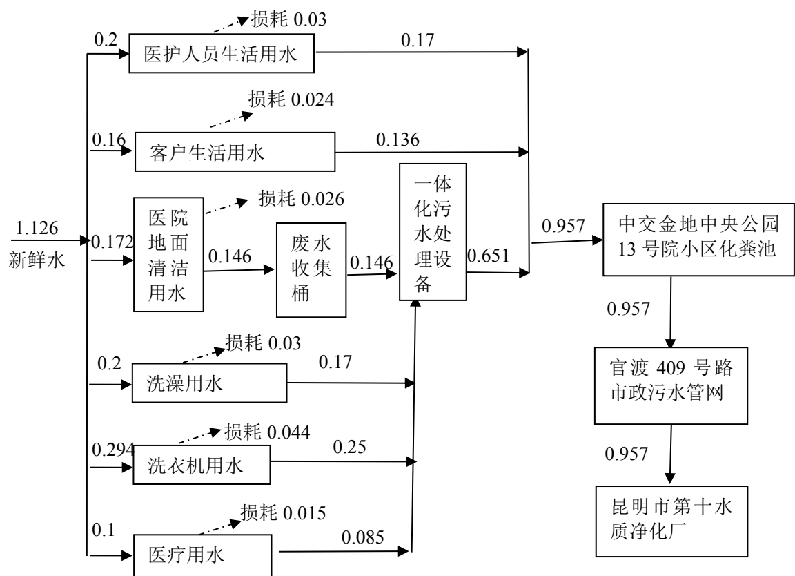
图 4-1 项目水平衡图 单位: m 3 /d
